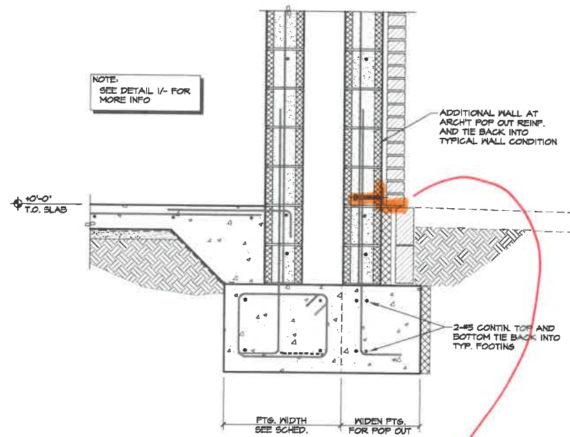
5 DETAIL SCALE: 1" = 1'-0"
