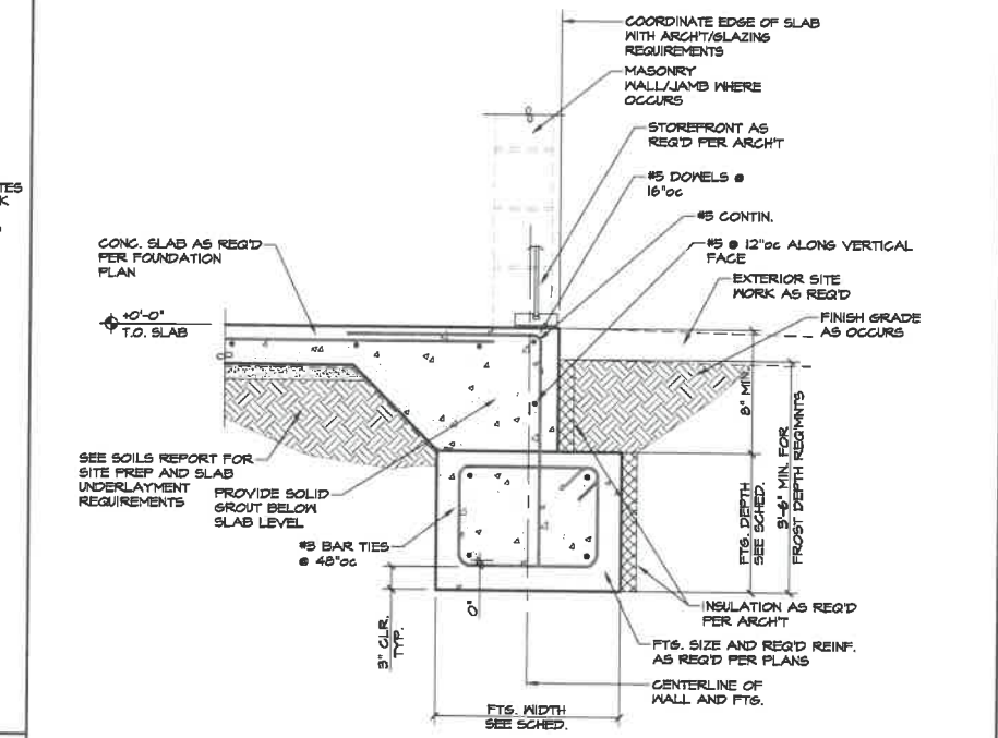
1 DETAIL SCALE: 1" = 1'-0"
