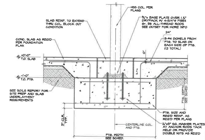
3 DETAIL SCALE: 1" = 1'-0"
